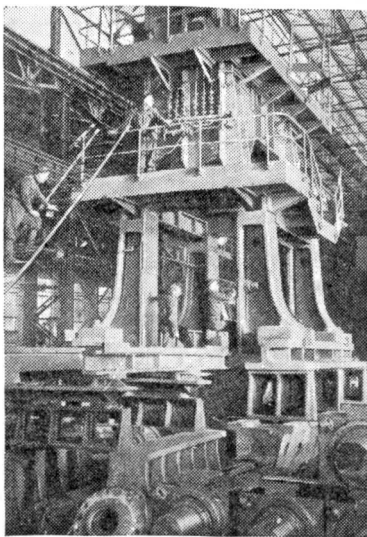
Свердловск. На Уральском заводе тяжелого машиностроения изготавливаются агрегаты для непрерывно-заготовочных (прокатных) станов, предназначенные для Польши и Китая.
