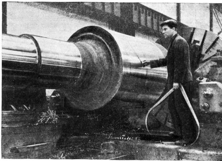
Ново-Краматорский завод на Украине по заказу польской промышленности изготавливает опорные валки для прокатного стана.
