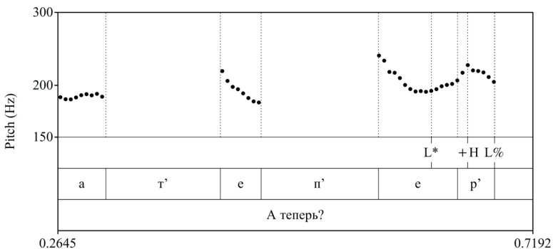
Рис. 9. Кривая ЧОТ общего вопроса А теперь? (ЛФ1932)
