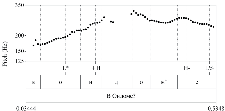
Рис. 10. Кривая ЧОТ общего вопроса В Ондоме? (МЯК1931)
