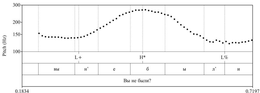
Рис. 18. Кривая ЧОТ общего вопроса Вы не были? (ТИК1943)
