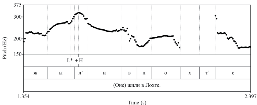
Рис. 27. Кривая ЧОГ: (Оне) жили в Лохте. (ЕКР1930)
