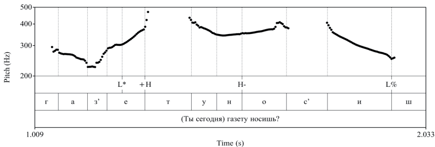
Рис. 1. Кривая ЧОТ общего вопроса Ты сегодня газету носишь? (АИ)
