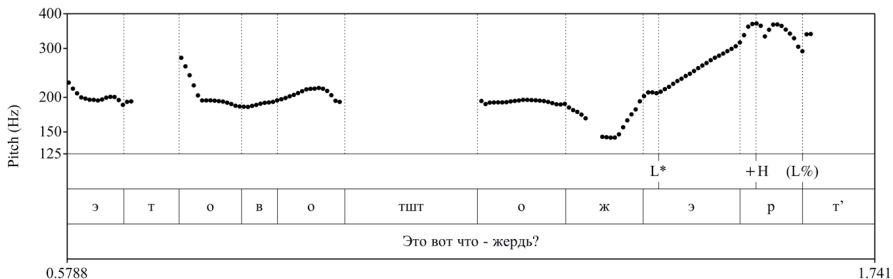
Рис. 7. Кривая ЧОТ общего вопроса Это вот что — жердь? (ЛФ1932)
