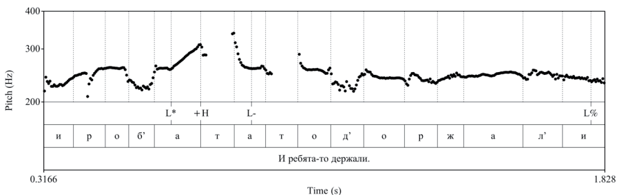
Рис. 20. Кривая ЧОТ: И ребята-то держали... (ЛФ1932)
