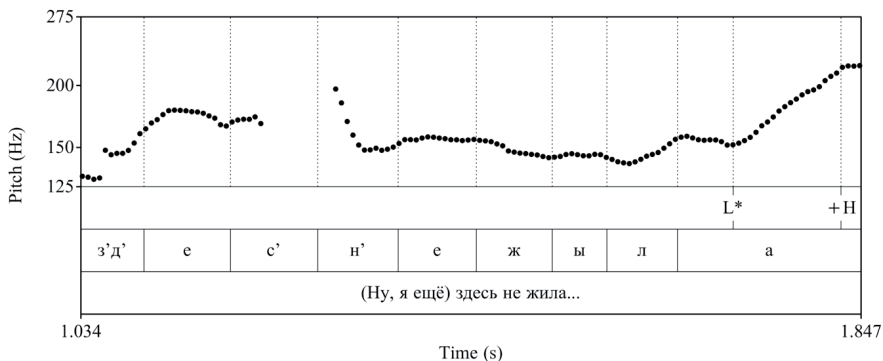
Рис. 26. Кривая ЧОГ: (Ну, я ещё) здесь не жила... (МЯК1931)
