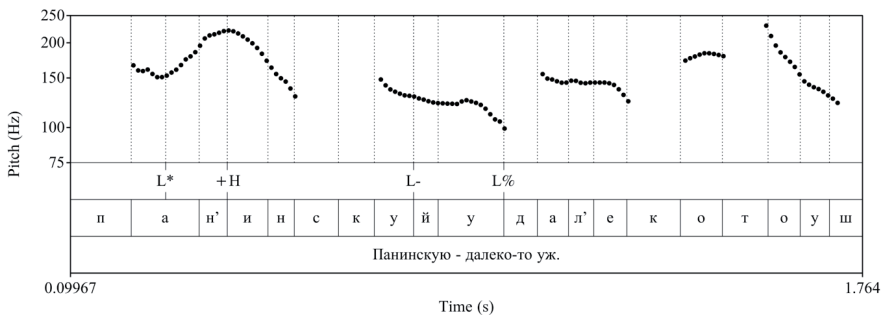
Рис. 25. Кривая ЧОГ: Панинскую — далеко-то уж. (АИ)
