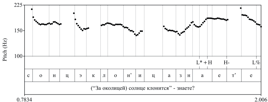
Рис. 14. Кривая ЧОТ общего вопроса Знаете? (ЕКТ1925)
