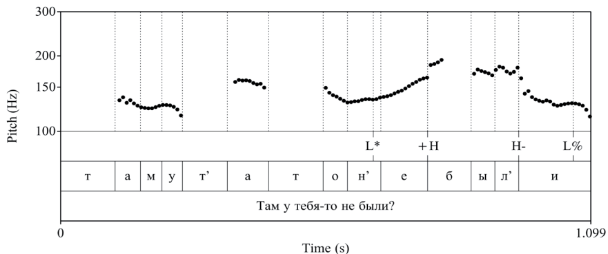
Рис. 3. Кривая ЧОТ общего вопроса Там у тебя-то не были? (АИ)
