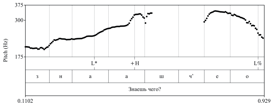
Рис. 12. Кривая ЧОТ общего вопроса Знаешь чего? (МЯК1931)
