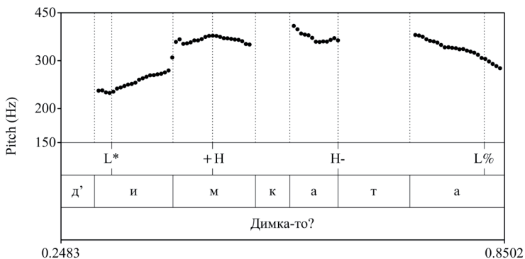
Рис. 11. Кривая ЧОТ общего вопроса Димка-то? (МЯК1931)
