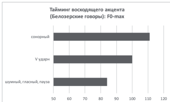
Рис. 32. Длительность отрезка ударного гласного акцентоносителя до точки максимума ЧОТ в процентах от общей длительности ударного гласного в зависимости от последующего сегмента
