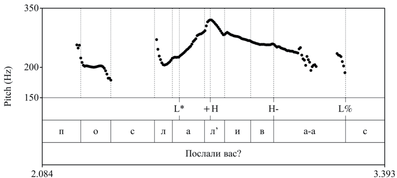
Рис. 6. Кривая ЧОТ общего вопроса Послали вас? (ЛФ1932)
