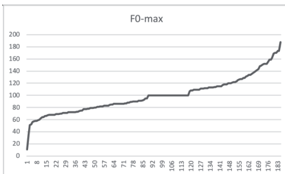
Рис. 33. Длительность отрезка ударного гласного акцентоносителя до точки максимума ЧОТ (F0-max) в процентах от общей длительности ударного гласного, все информанты
