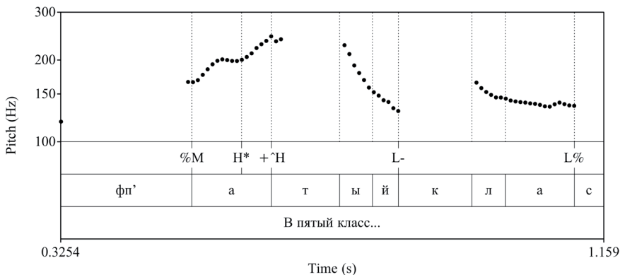
Рис. 22. Кривая ЧОТ: В пятый класс... (АИ)
