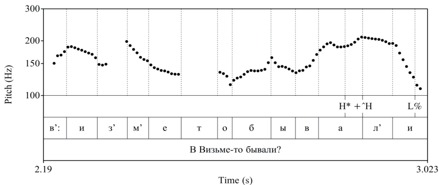
Рис. 2. Кривая ЧОТ общего вопроса В Визьме-то бывали? (АИ)
