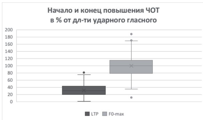
Рис. 35. Диаграмма размаха длительности отрезка ударного гласного акцентоносителя 1) до точки начала повышения тона (слева, LTP) и 2) до точки максимума ЧОТ (справа, F0-max) в процентах от общей длительности ударного гласного в общем вопросе
