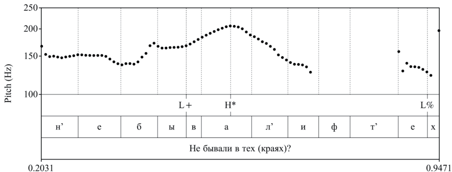
Рис. 4. Кривая ЧОТ общего вопроса Не бывали в тех (краях)? (АИ)
