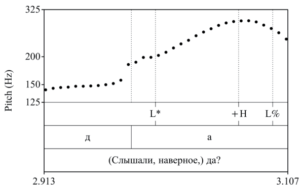
Рис. 17. Кривая ЧОТ общего вопроса да? (ТИК1943)
