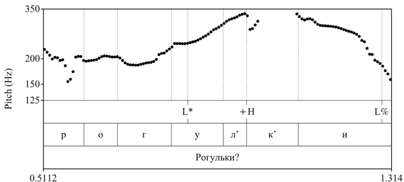
Рис. 5. Кривая ЧОТ общего вопроса Рогульки? (ЛФ1932)
