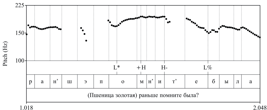
Рис. 15. Кривая ЧОТ общего вопроса раньше помните была? (ЕКТ1925)
