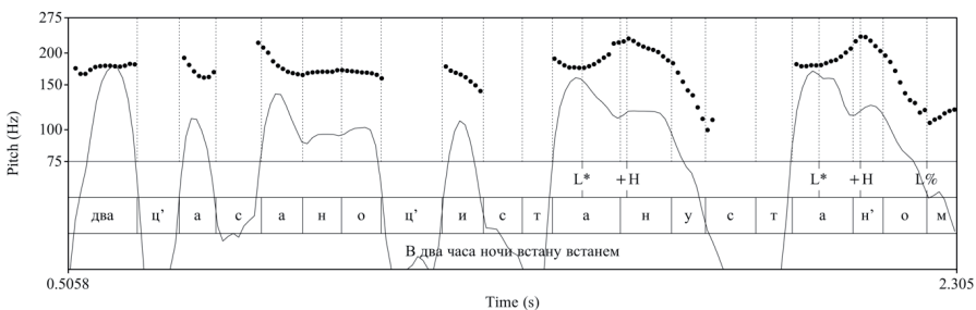
Рис. 24. Кривая ЧОТ и огибающая интенсивности: В два часа ночи встану... встанем... (АИ)
