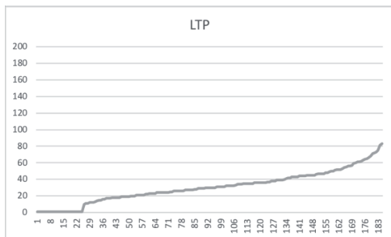
Рис. 34. Длительность отрезка ударного гласного акцентоносителя до точки начала повышения тона (LTP) в процентах от общей длительности ударного гласного, все информанты
