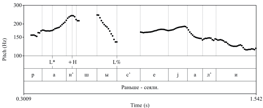
Рис. 23. Кривая ЧОТ: Раньше — сеяли. (АИ)
