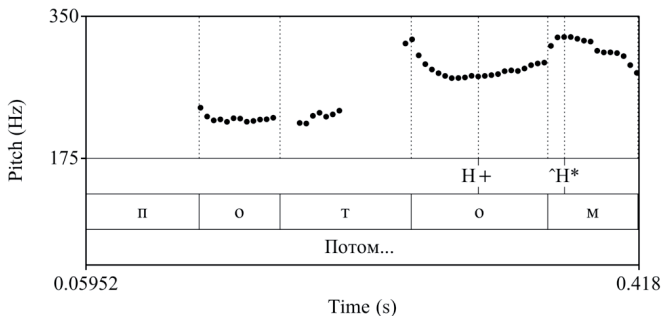
Рис. 28. Кривая ЧОТ: Потом... (ЕКР1930)
