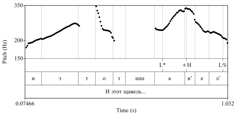
Рис. 21. Кривая ЧОТ: И этот щавель... (ЛФ1932)
