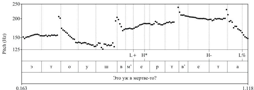
Рис. 16. Кривая ЧОТ общего вопроса Это уж в мертве-то? (ЕКТ1925)
