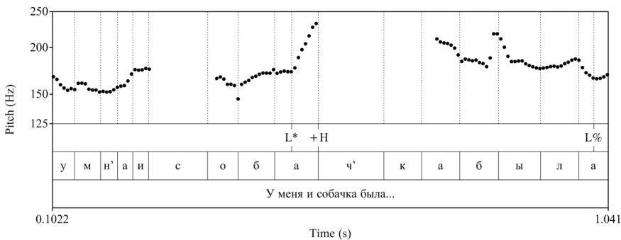
Рис. 30. Кривая ЧОТ: У меня и собачка была... (ЕКР1930)
