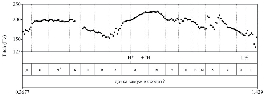
Рис. 13. Кривая ЧОТ общего вопроса Дочка замуж выходит? (ЕКТ1925)
