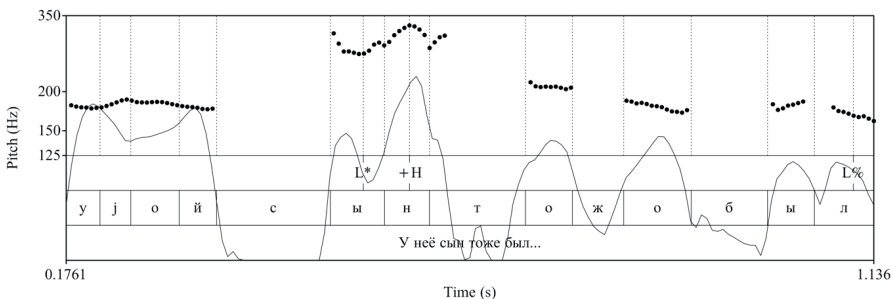
Рис. 29. Кривая ЧОТ и огибающая интенсивности: У неё сын тоже был... (ЕКР1930)
