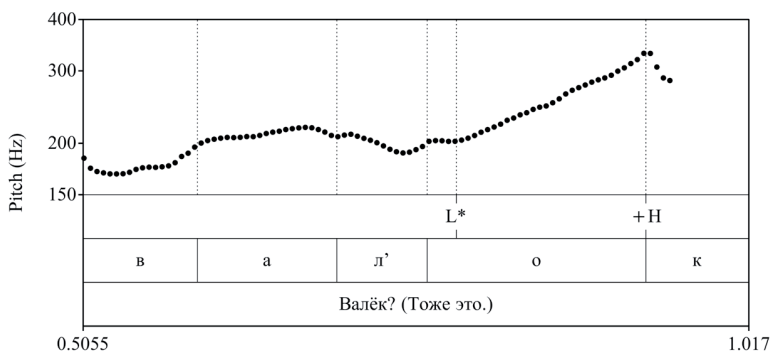
Рис. 8. Кривая ЧОТ общего вопроса Валёк? (Тоже это.) (ЛФ1932)
