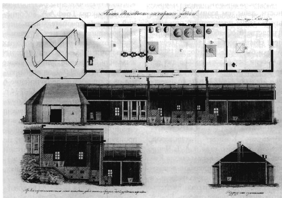
План сахарного завода И.А. Мальцова
